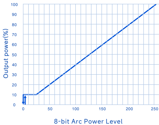
Linear Dimming Curve:(DALI-2 Model
